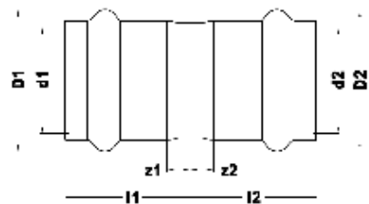
Fig. 3: Dimensions (Example DN20) d1 = 22 mm; D1 = 31 mm l1, l2 = 29 mm; z1, z2 = 6 mm
